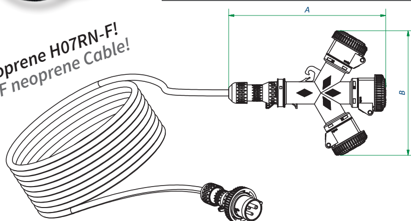
DIMENSIONI - SIZES
